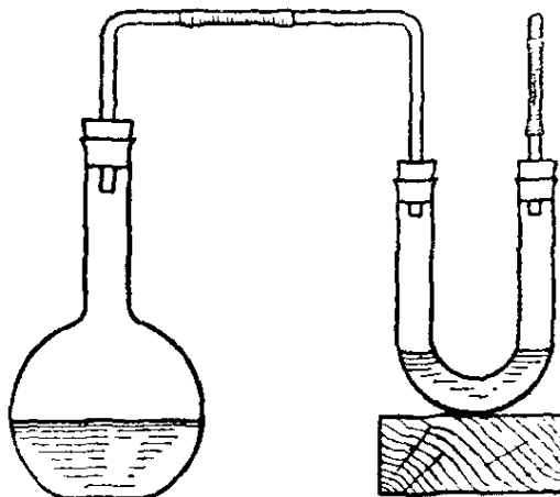
Рис. 1. Брожение глюкозы.
