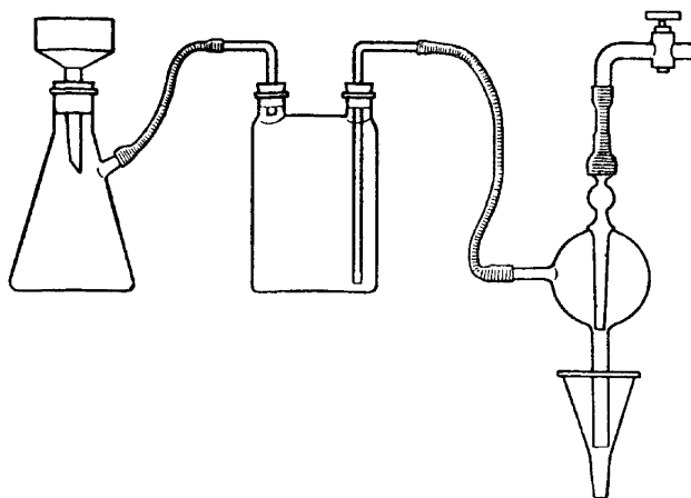
Рис. 2. Фильтровальная установка.
